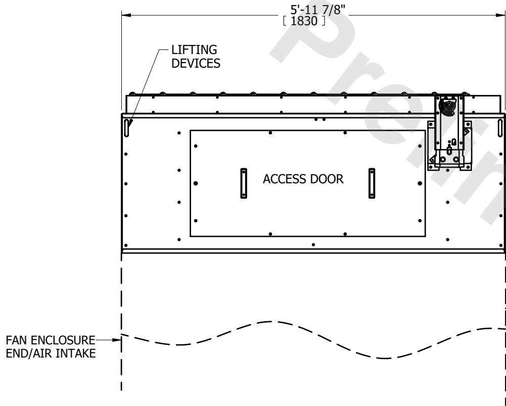
FACE C
