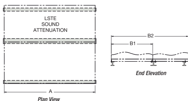
LSTE DIMENSIONS
