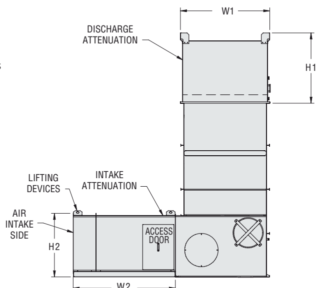
LSTE Attenuation
