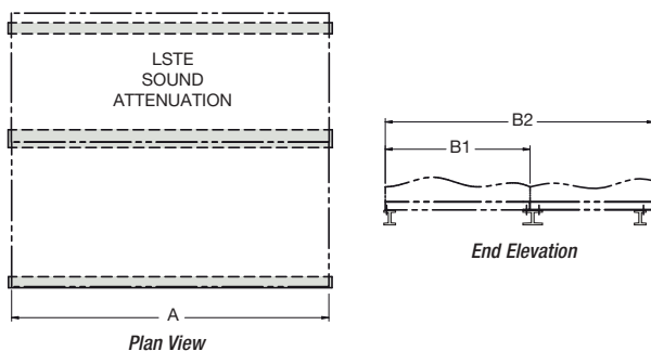
LSTE DIMENSIONS
