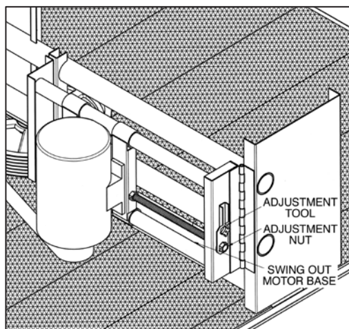
Figur 4 - Invändigt monterad motor, kylfläkt
