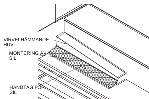
Figur 12 - Montering av PHC-SE-filter
