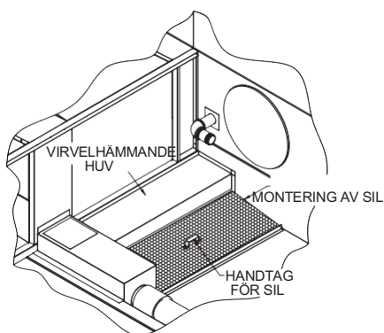
Figur 11 - LRWB/LRC-montering av sil
