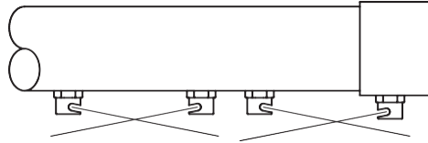
Figur 16 - Korrekt orientering av vattenspridare (2A-munstycken) - ESW4-modeller
