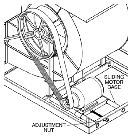
Figur 8 - Justering av LR-motor
