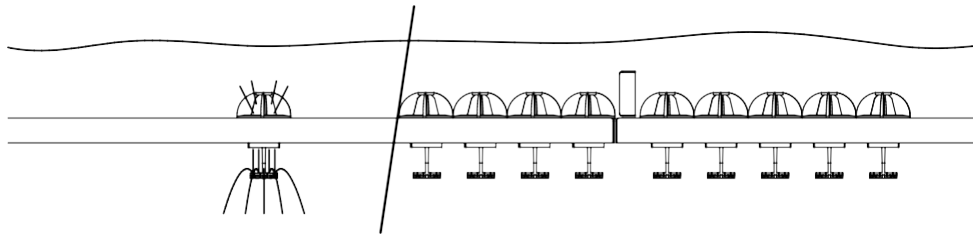
Figur 18 - Gravitationsmatad fördelningslåda - endast ESW4-modeller
