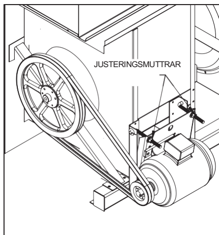
Figur 7b - Externt monterad motor, små LS-, 4X- och 5X-enheter
