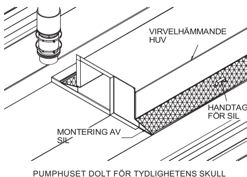
Figur 13 - Montering av PHC-DE-filter
